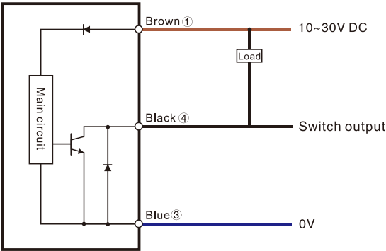
NPN Output
