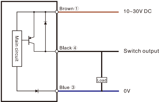
PNP Output
