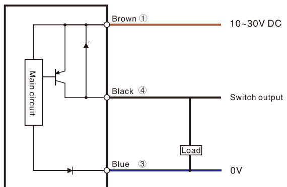
PNP Output
